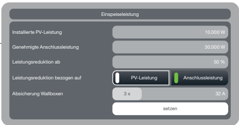
Beispiel: Einstellung einer 22 kW Wallbox auf 30 kW Hausmaximaleistung mit 10 kW PV-Anlage
